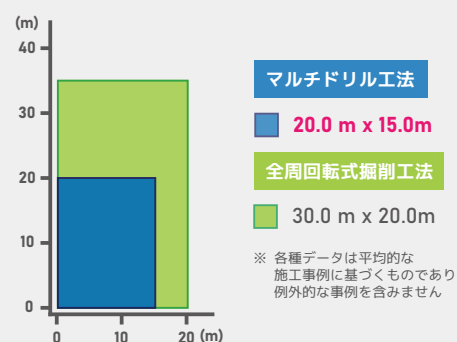
標準施工ヤードの比較
