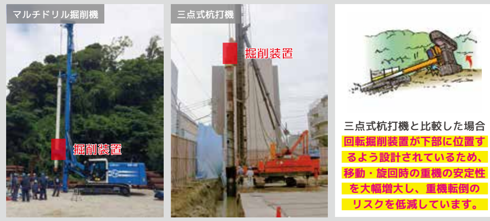
三点式杭打機との掘削装置位置の比較
