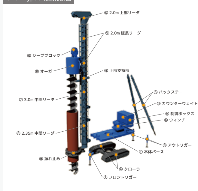
OTO®-Type 3 機械分解図
